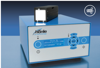
LED Spot 40 IC kompakter Flächenstrahler mit hohen Intensitäten
